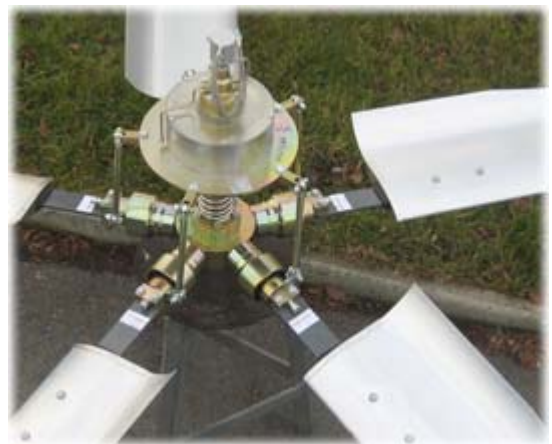
5 bladed flexy AV fan
